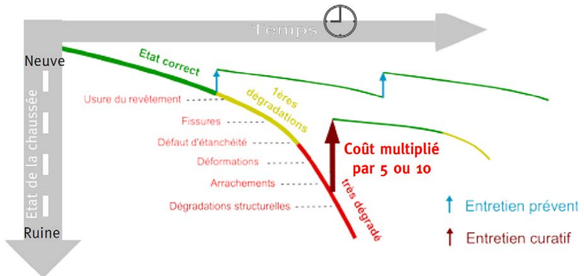
Graphique 5 : Schéma de dégradation d'une route
